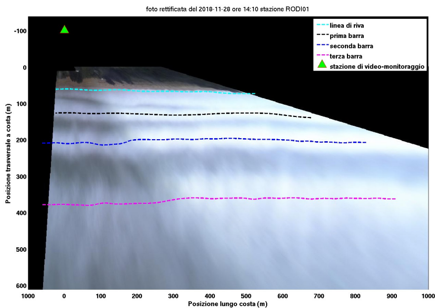
Figura 21. Visione orto-rettificata della spiaggia di Rodi Garganico.
