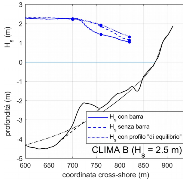
Figura 36. Andamento dell'altezza significativa H_s sulle tre batimetrie di figura 34 per clima ondoso moderato ( H_s = 2.5 m al largo). I pallini indicano la posizione dei tre punti significativi a cui fanno riferimento i valori della Tabella 4 ( x = 700, 760, 820 m)
