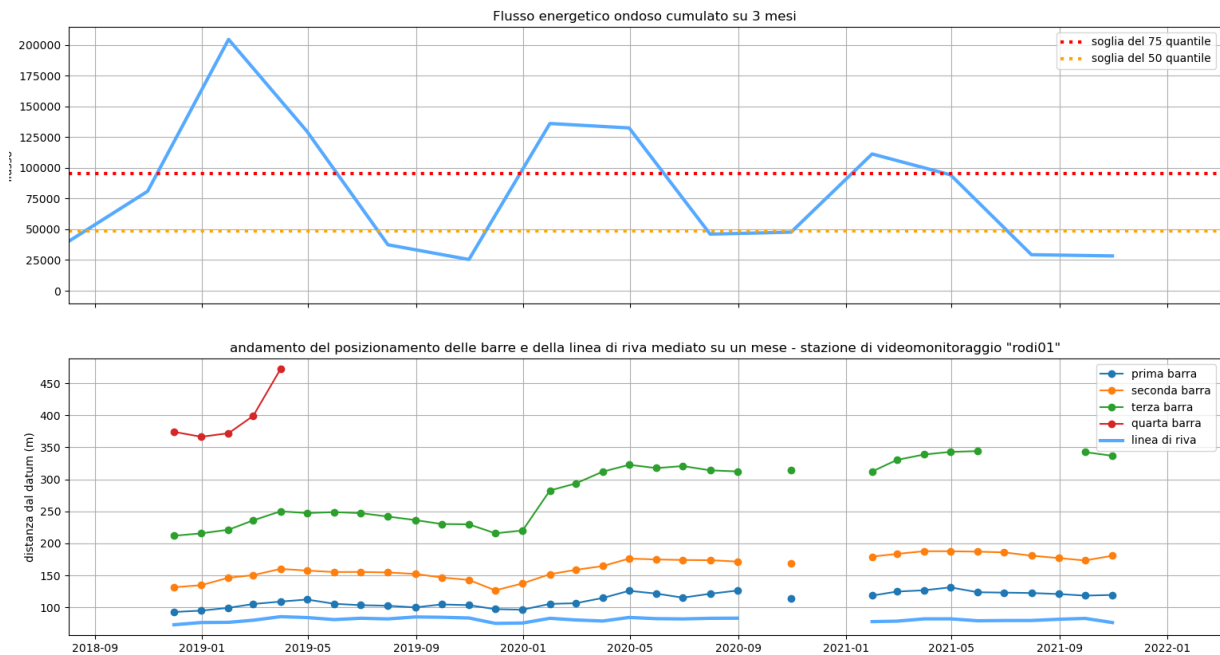
Figura 22. Pannello superiore: flusso energetico ondoso cumulato trimestralmente; Pannello inferiore: evoluzione del sistema spiaggia di Rodi Garganico desunto da dati di videomonitoraggio.
