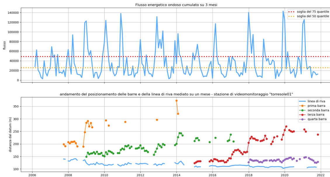
Figura 15. Pannello superiore: flusso energetico ondoso cumulato trimestralmente; Pannello inferiore: evoluzione del sistema spiaggia di Terracina desunto da dati di video-monitoraggio.
