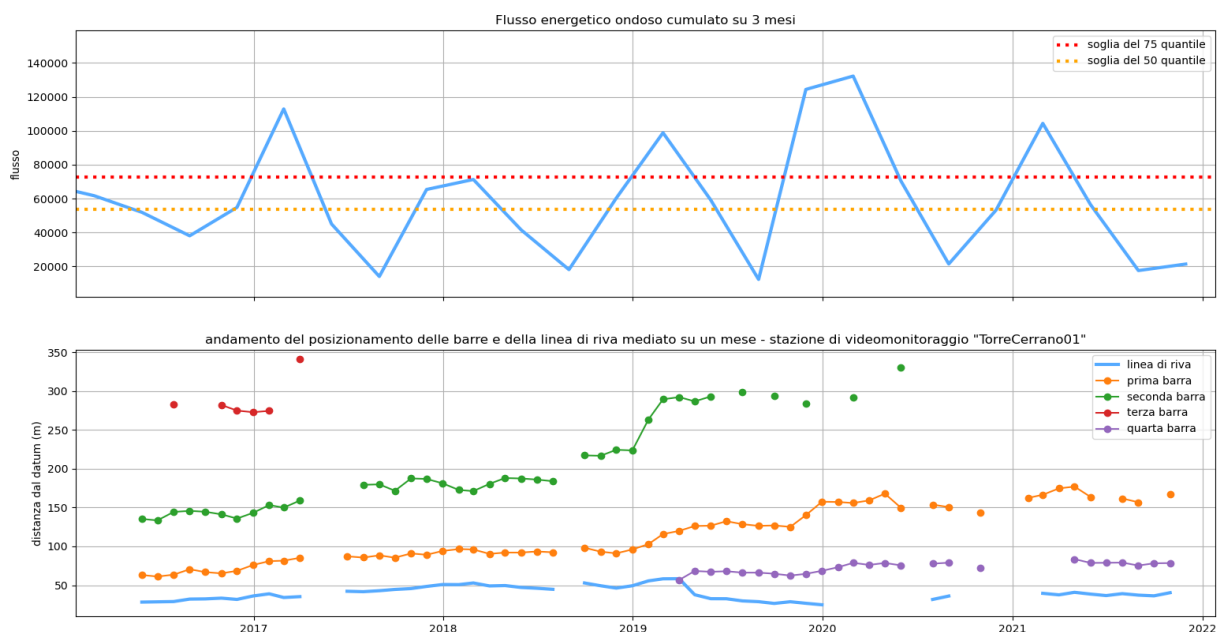
Figura 26. Pannello superiore: flusso energetico ondoso cumulato trimestralmente; Pannello inferiore: evoluzione del sistema spiaggia di Torre del Cerrano desunto da dati di videomonitoraggio.
