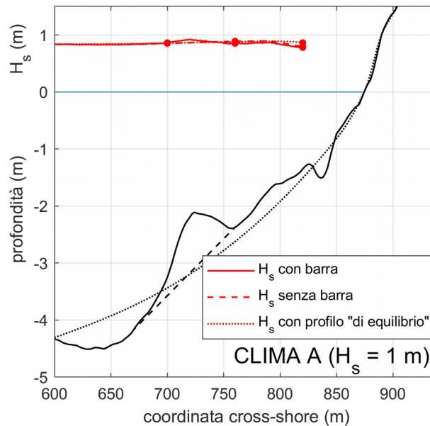
Figura 35. Andamento dell'altezza significativa H_s sulle tre batimetrie di figura 34 per clima ondoso poco intenso ( H_s = 1 m al largo). I pallini indicano la posizione dei tre punti significativi a cui fanno riferimento i valori della Tabella 4 ( x = 700, 760, 820 m)
