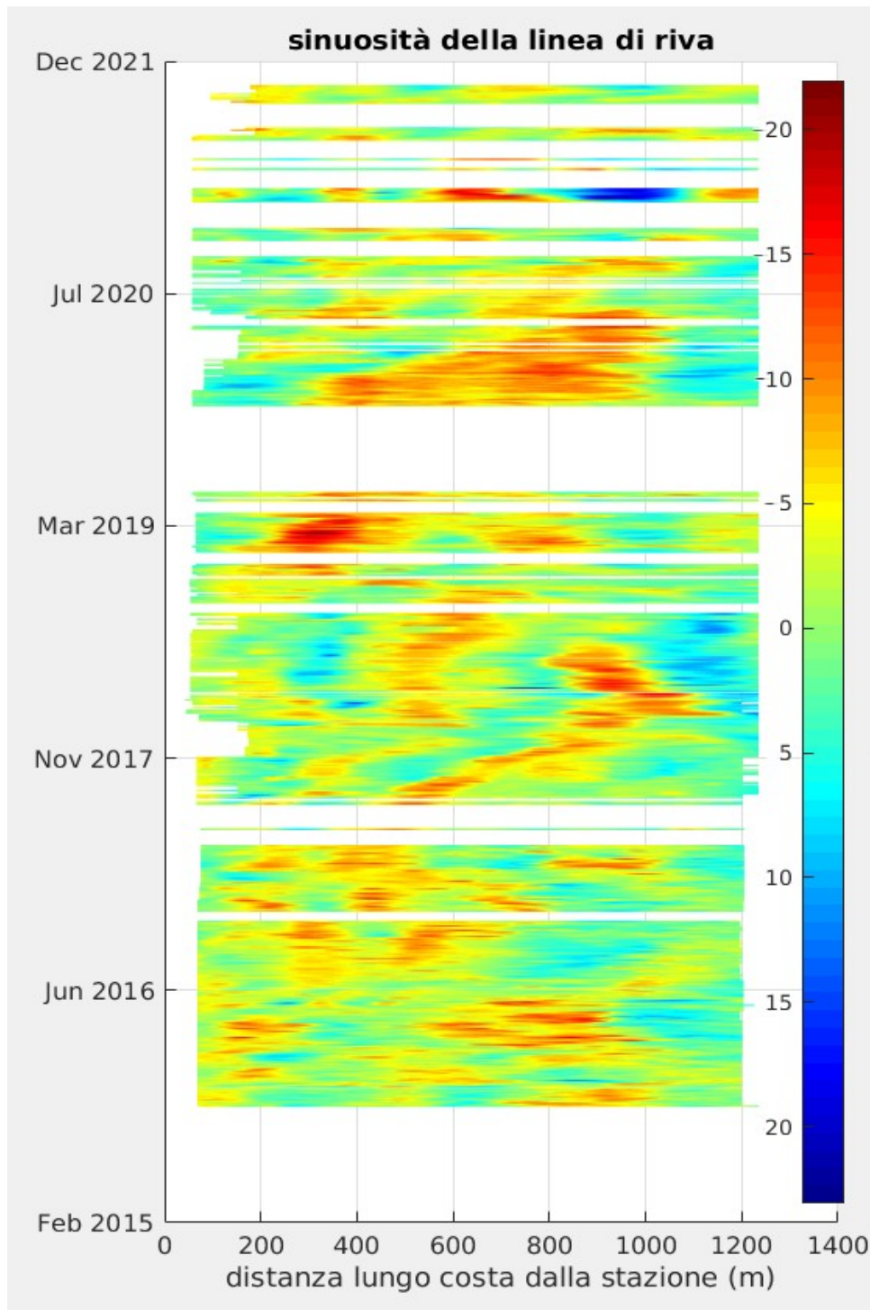
Figura 12. Andamento della sinuosità della linea di riva, ovvero ampiezza delle cuspidi (colore blu) e delle baie (colore rosso) lungo il tratto analizzato [dalla stazione Kufra sino a 1200m verso sud].
