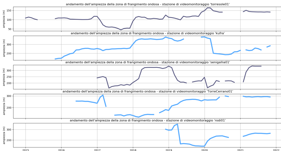
Figura 32. Andamento temporale dell'ampiezza della zona dei frangenti per le aree analizzate (in blu). Per confronto si riporta il valore computato sui litorali di Terracina e Senigallia (in grigio).
