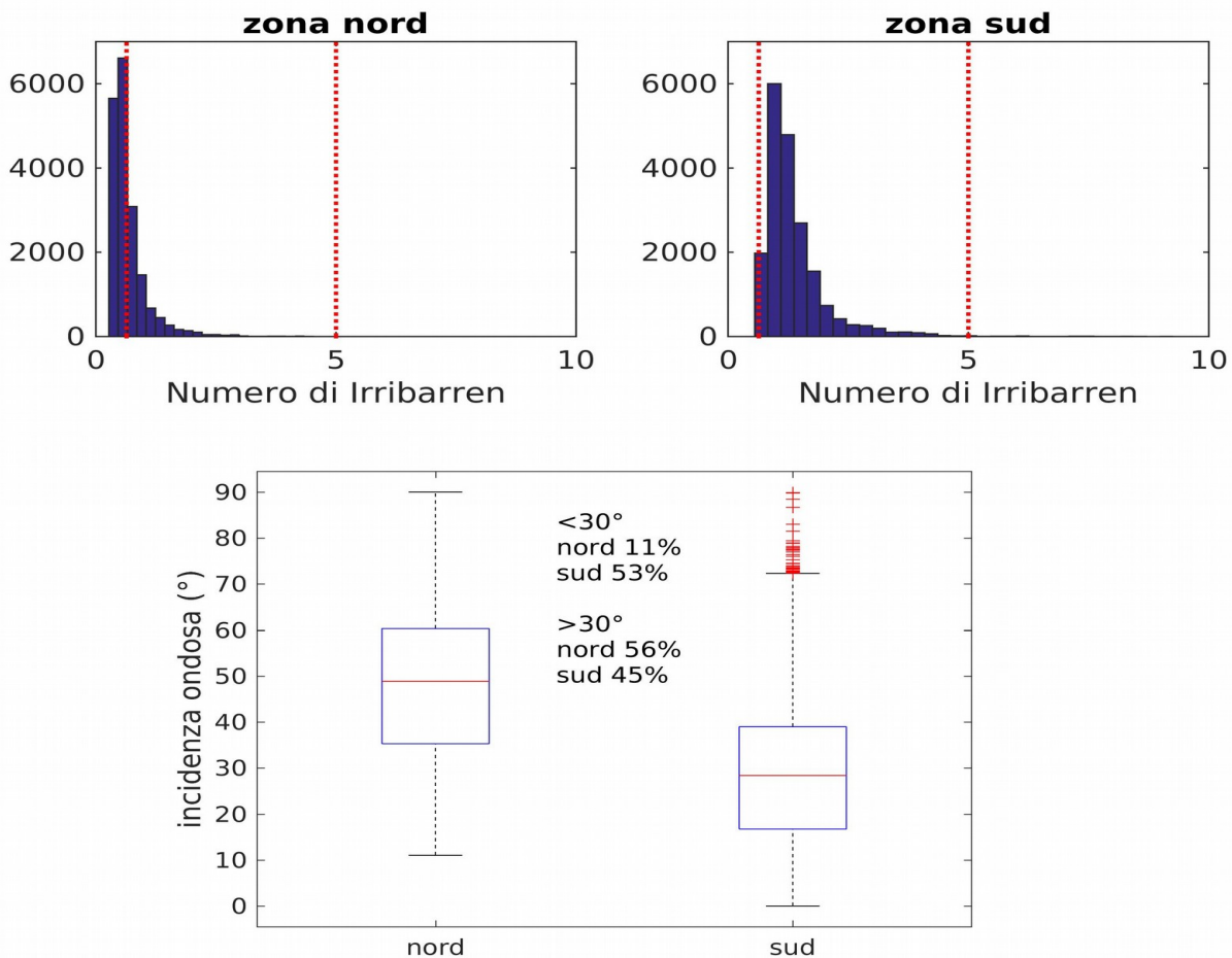
Figura 8. Pannelli superiori indicanti la distribuzione statistica del parametro di Irribarren in funzione di una serie temporale di 10 anni di dati ondometrici estratti dalla boa virtuale antistante il litorale del PNC, le linee rosse indicano le soglie tra tre stadi morfodinamici. Nel pannello inferiore la distribuzione statistica dell'obliquità ondosa calcolata per le due aree.
