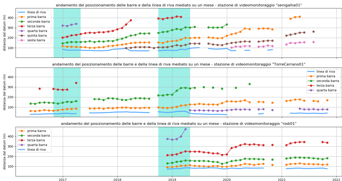
Figura 30. Andamento dell'assetto morfologico dei fondali con specifico riferimento a due intervalli temporali contraddistinti da elevato valore dell'energia ondosa (zone ciano).
