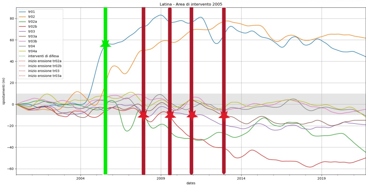
Figura 19. Descrizione dell'evoluzione temporale del fenomeno erosivo/deposizionale nell'intorno della zona soggetta a intervento di difesa 2003-2004 costituito da ripascimento e costruzione di pennelli trasversali e barriere soffolte. La banda grigia rappresenta la soglia di risoluzione massima del dato, ovvero 10m.
