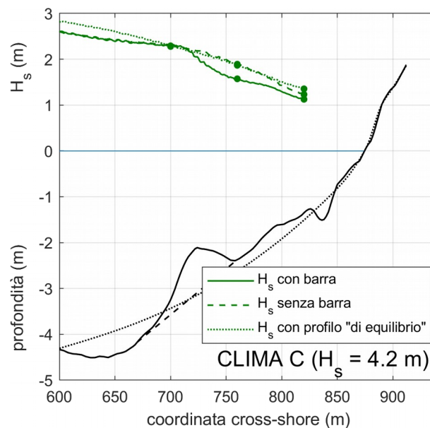
Figura 37. Andamento dell'altezza significativa H_s sulle tre batimetrie di figura 34 per clima ondoso intenso ( H_s = 4.2 m al largo). I pallini indicano la posizione dei tre punti significativi a cui fanno riferimento i valori della Tabella 4 ( x = 700, 760, 820 m)
