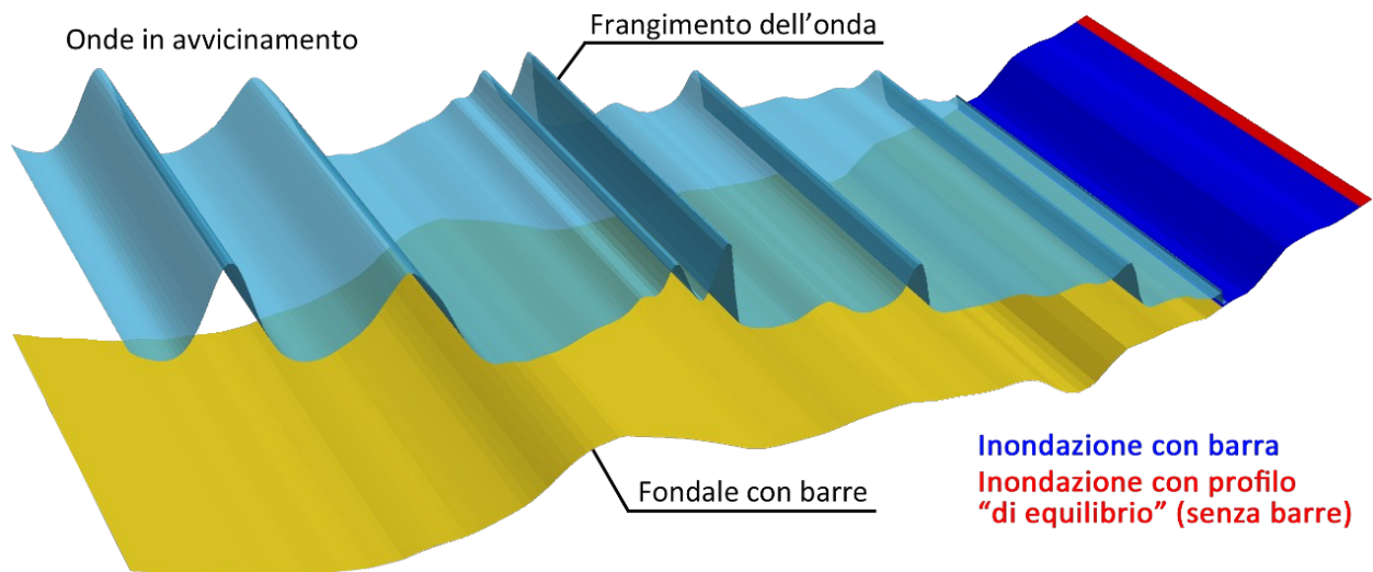
Figura 38. Rappresentazione grafica dei processi di trasformazione dell'onda e dell'inondazione significativa per clima ondoso medio ( H_s = 2.5 m). In blu è indicata l'inondazione significativa del profilo con barra; in rosso quella del profilo "di equilibrio". Nota: la scala verticale è esasperata rispetto a quella orizzontale.
