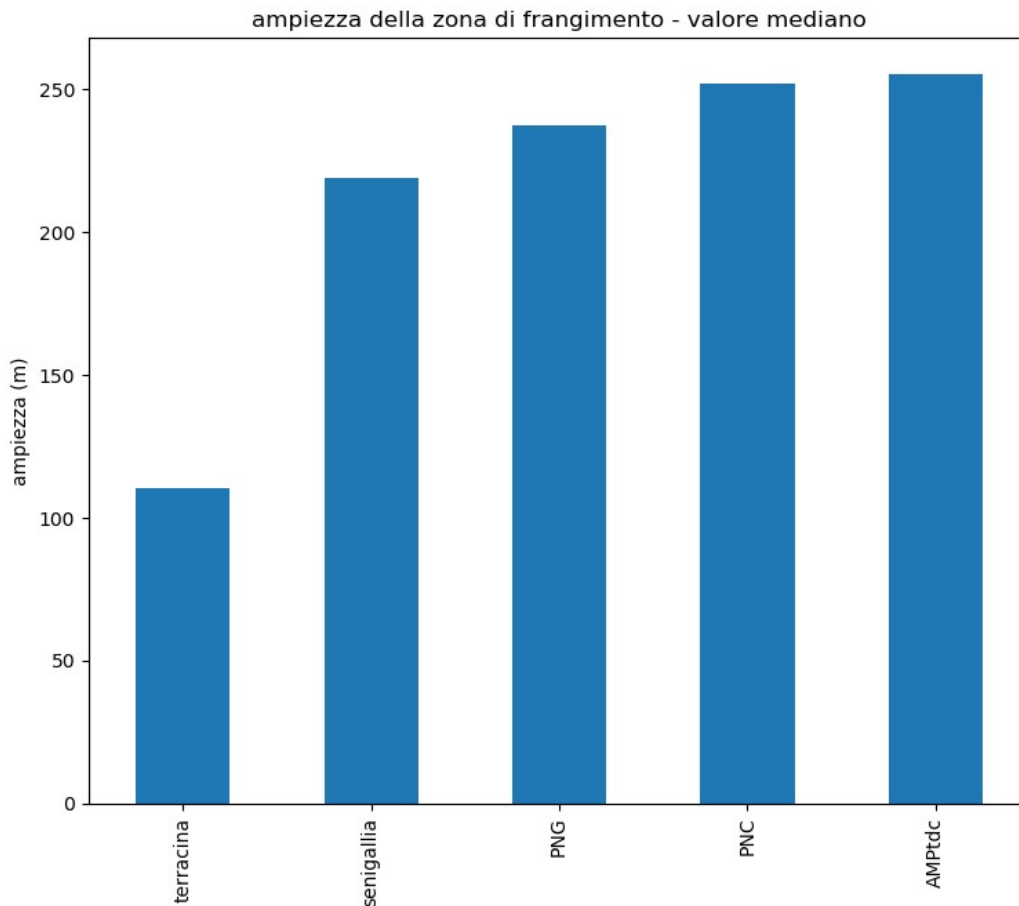
Figura 29. Ampiezza della zona dei frangenti per le aree analizzate. Per confronto si riporta il valore computato sui litorali di Terracina e Senigallia.
