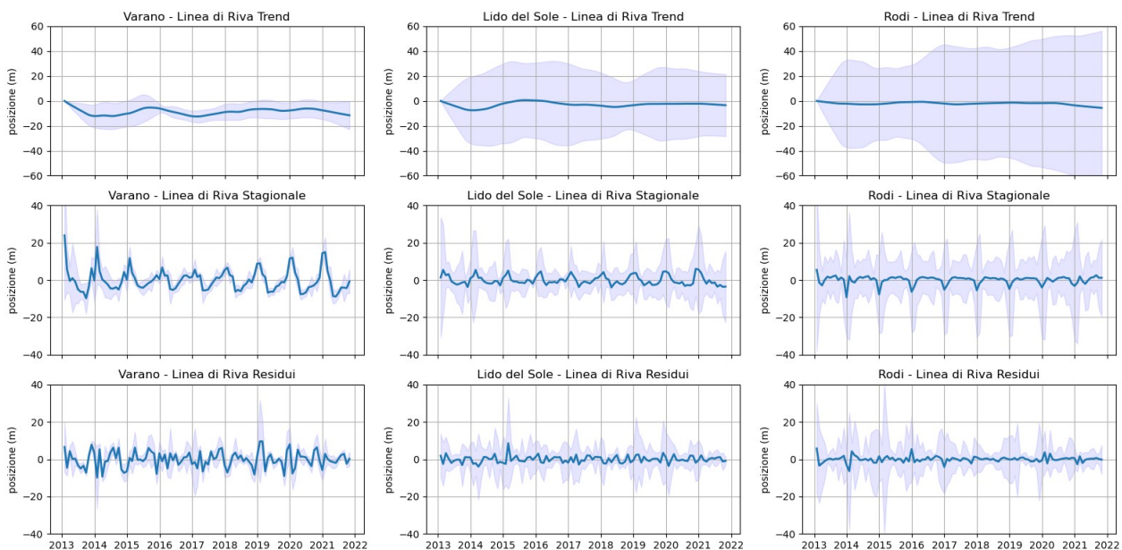
Figura 24. Andamento della linea di riva e rispettivi componenti per le tre sub-unità del PNG.
