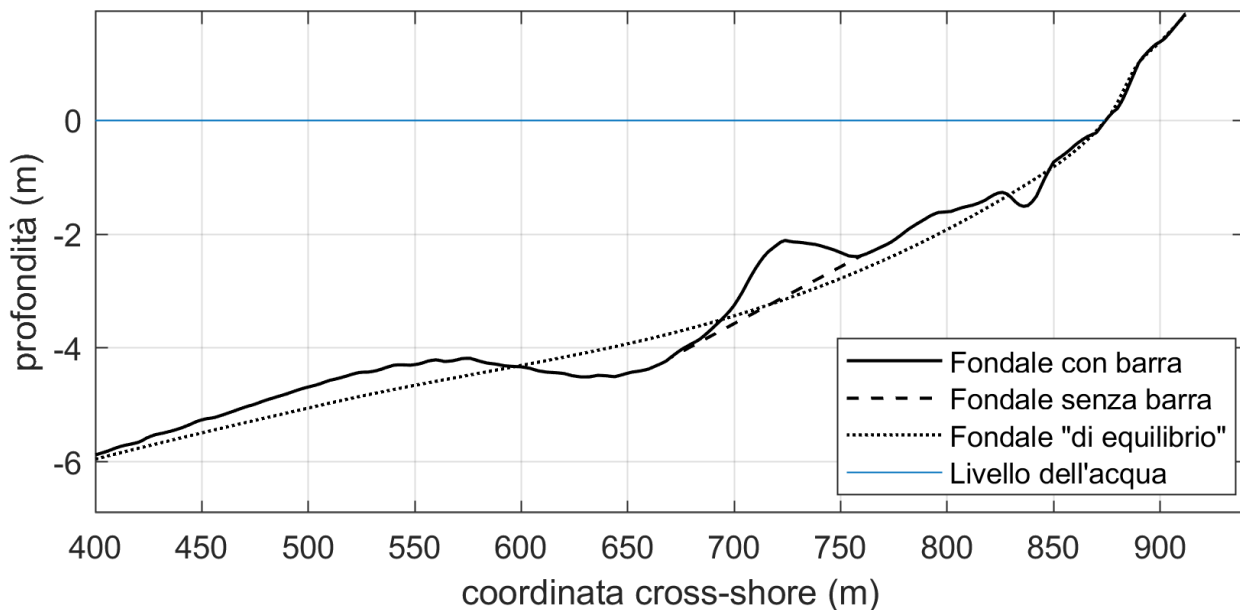
Figura 34. I tre profili utilizzati per le simulazioni di valutazione dell'effetto delle barre sottomarine.
