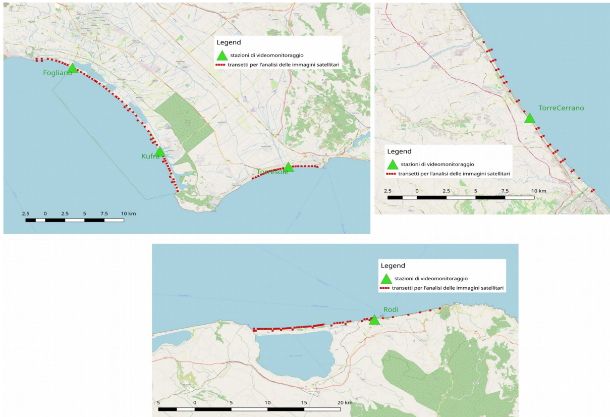
Figura 6. Localizzazione dei transetti di misura del posizionamento della linea di riva estratto da immagini multispettrali satellitari.
