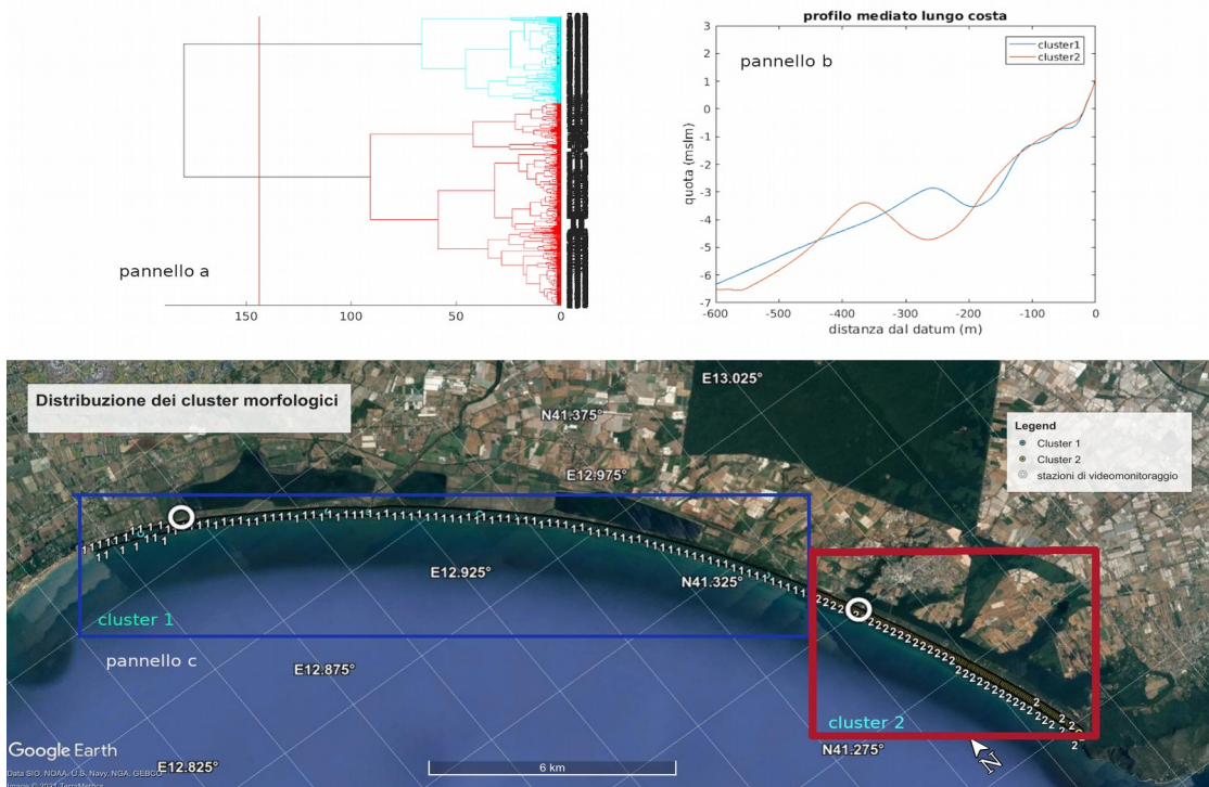
Figura 7. Cluster morfologici che descrivono il comportamento del litorale del PNC.
