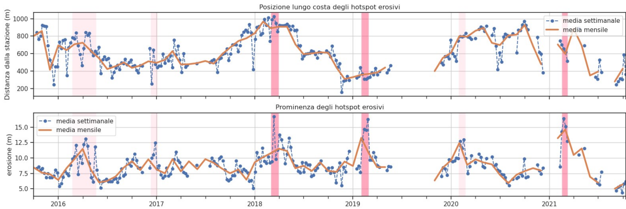
Figura 13. Andamento dei fenomeni erosivi dovuti alle cuspidi. Nel pannello superiore la localizzazione lungo costa dei fenomeni erosivi, nel pannello inferiore l'entità dell'erosione. In rosso chiaro gli eventi con erosione della spiaggia maggiore di 15m, in rosa gli eventi con erosione minore di 15m.
