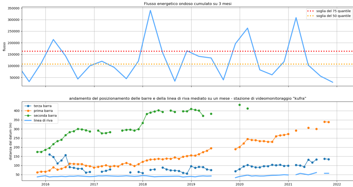
Figura 14. Pannello superiore: flusso energetico ondoso cumulato trimestralmente; Pannello inferiore: evoluzione del sistema spiaggia di Sabaudia desunto da dati di video-monitoraggio.
