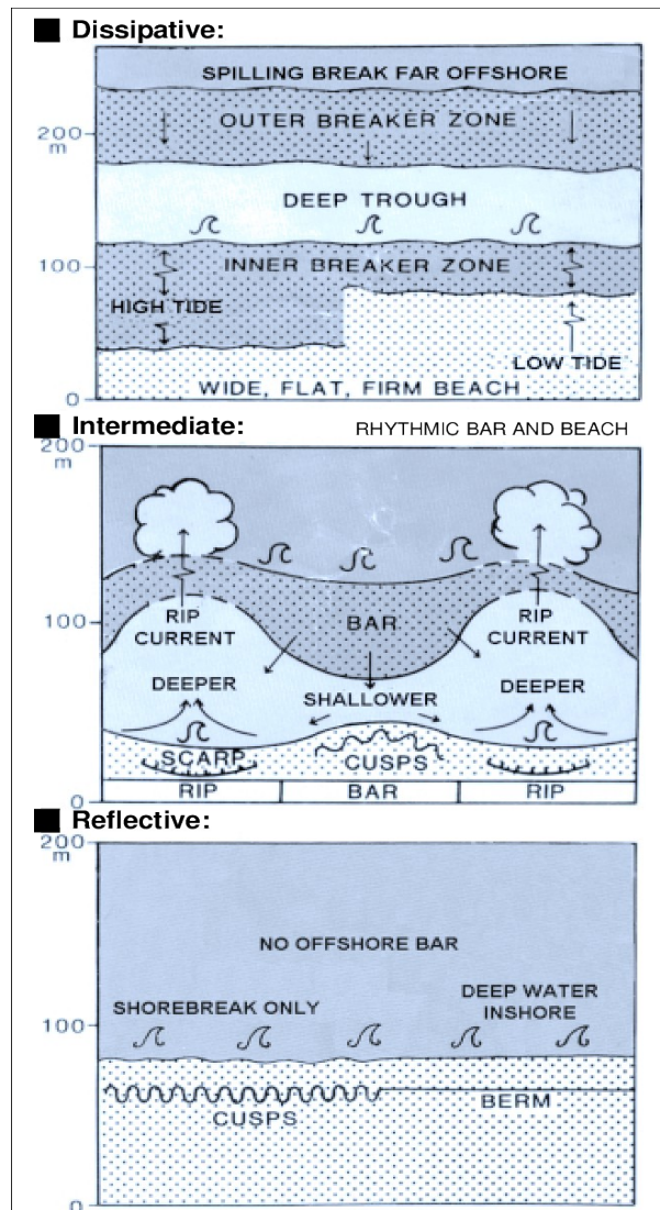
Figura 10. Schema concettuale del modello morfodinamico di Wright & Short.
