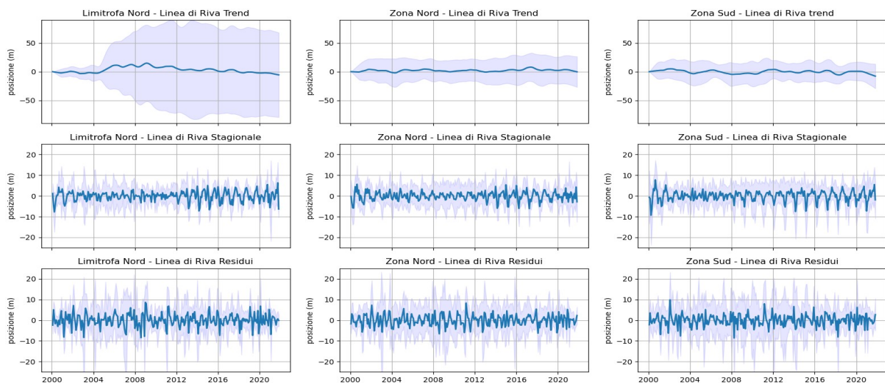
Figura 18. Andamento della linea di riva e rispettivi componenti per le tre sub-unità del PNC.
